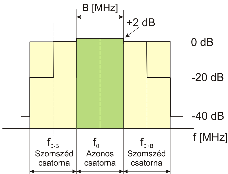
18. ábra. A Hírközlési hatóság ajánlása interferencia számításához
