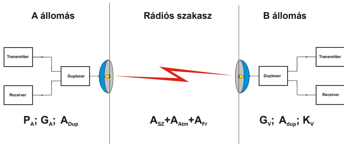
13. ábra. A szakasz számítás elemei
