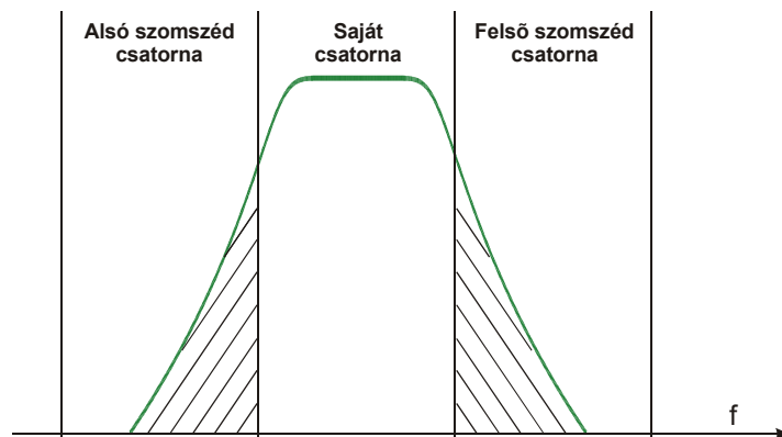
17. ábra. Csatorna elhelyezkedés és szűrő karakterisztika
